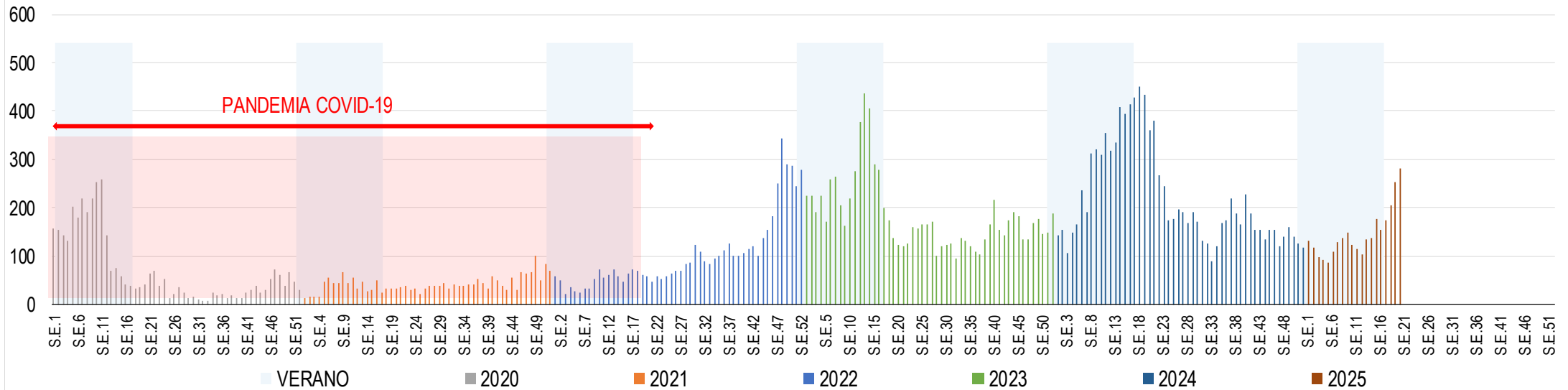
CURVA EPIDEMICA DE FEBRILES (2019 HASTA 2024 (AÑOS CERRADOS) Y 2025 A LA S.E.20)
