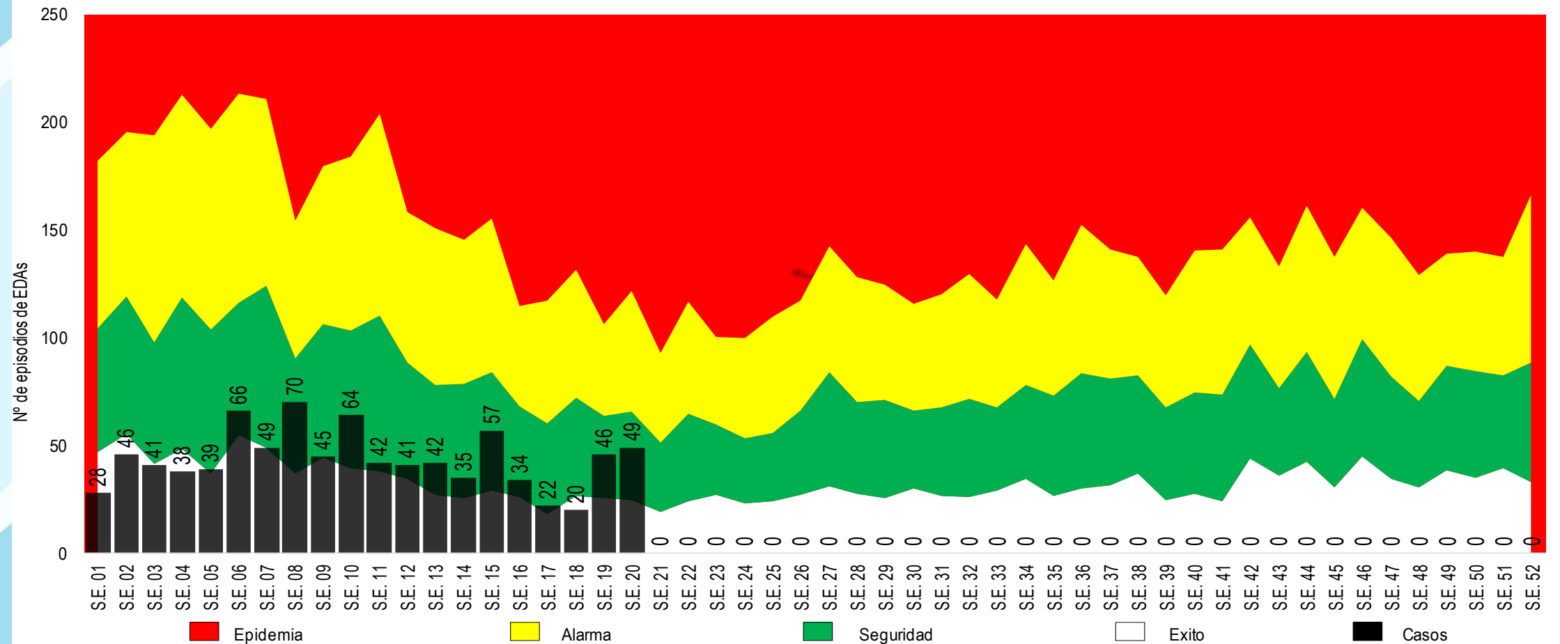
CANAL ENDÉMICO DE CASOS NOTIFICADOS POR EDA's A LA S.E. N° 20 - 2025 HOSPITAL REGIONAL HUACHO
