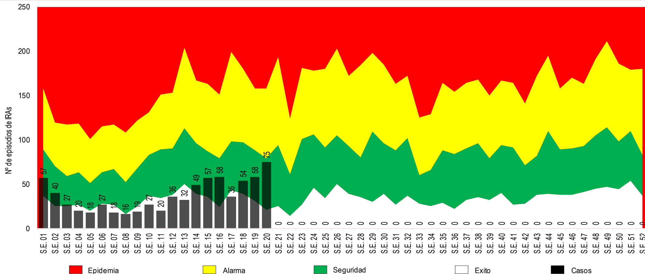
CANAL ENDÉMICO DE CASOS NOTIFICADOS POR IRA's A LA S.E. N° 20 - 2025 HOSPITAL GENERAL HUACHO
